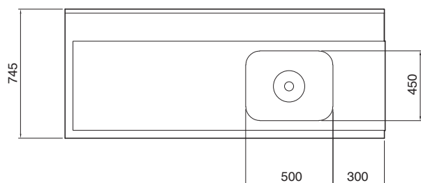
Planta
